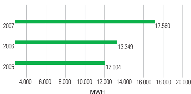
Κατανάλωση ηλεκτρικής ενέργειας μεγάλων κτηρίων
